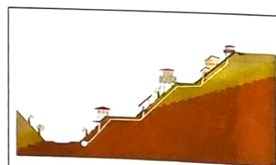
Figura 4 – Esquema de solução em encosta – coleta total
